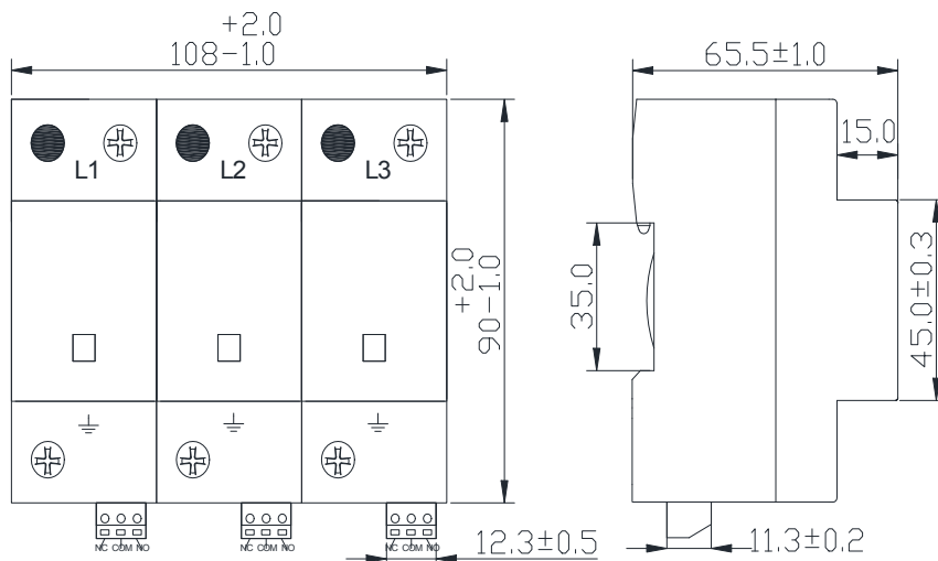
图 4-1 RPM1400-30/3P 外形尺寸图
