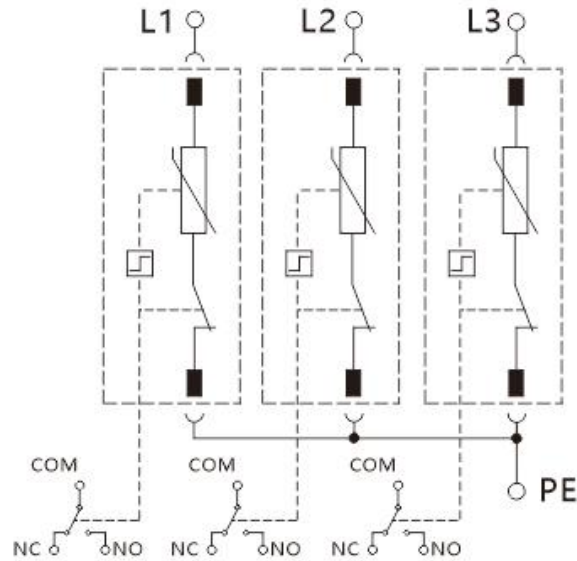
图 3-1 RPM1400-30/3P 三相电源模块式浪涌保护器 保护原理示意图
